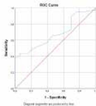
ROC Eğrisi
